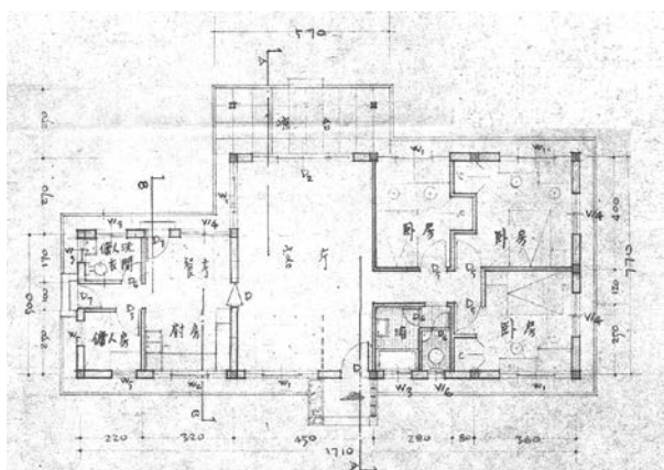
圖8：1966年新建的乙種宿舍單元平面圖（成大營繕組檔案）。
