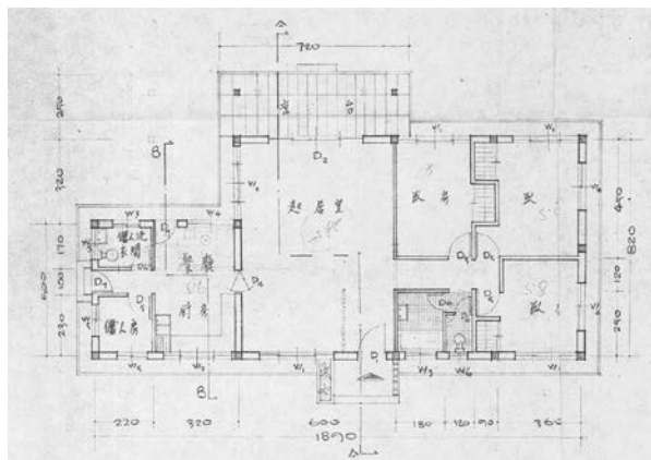
圖9：1966年新建的甲種宿舍單元平面圖（成大營繕組檔案）。
