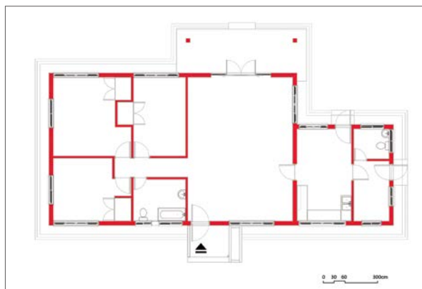
圖10：大學路22巷27號測繪平面圖（李柏霖2022年繪製）。
